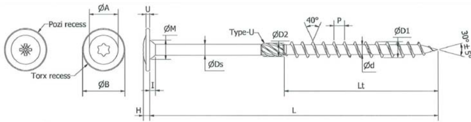
Type-17
