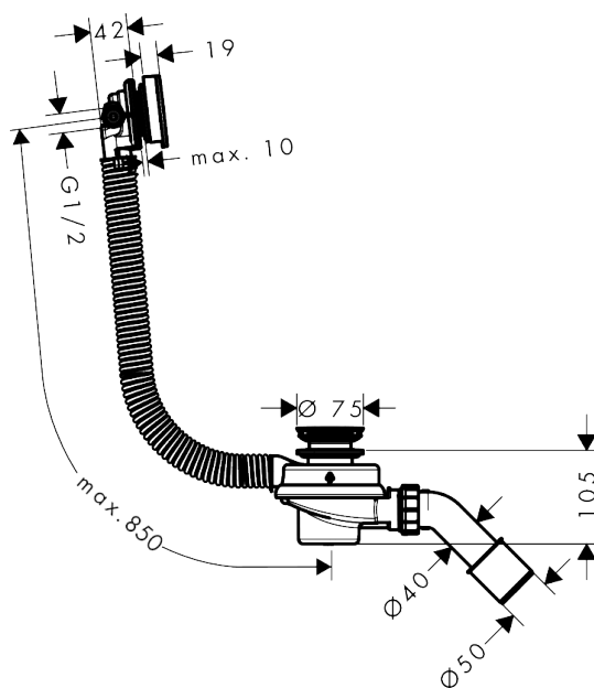
Maattekening
