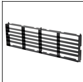
GWP30002 Lichtaafscherming voor versies met ronde optiek
