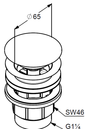
Maßzeichnung/ Dimensional drawing
