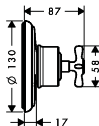
AXOR Citterio 39925XX0
