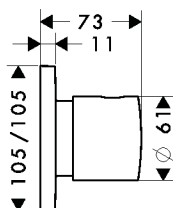
AXOR Citterio M 34920XX0
