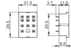
Aanzicht aansluitingen
