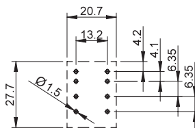
Aanzicht aansluitingen
