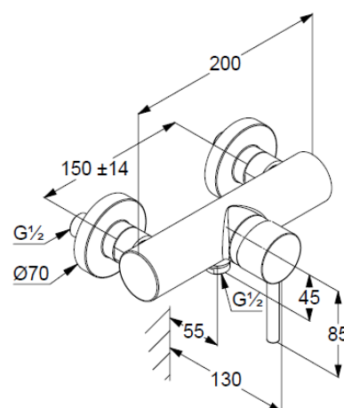
Maßzeichnung/ Dimensional drawing
