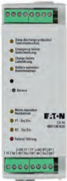
CG IV.1 relay module
