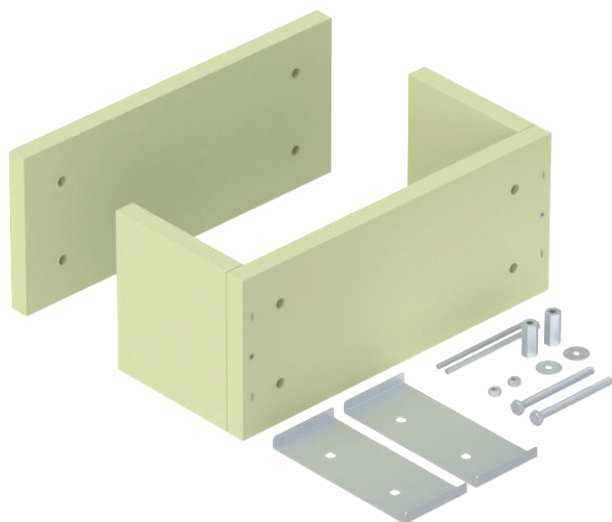
Calciumsilicaat
