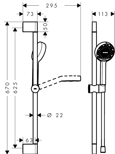
Maattekening
