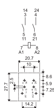
56.42-0300 Aanzicht op de aansluitingen
