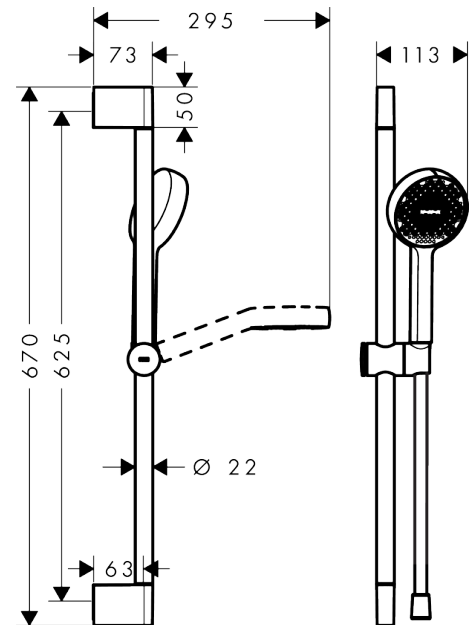
Maattekening
