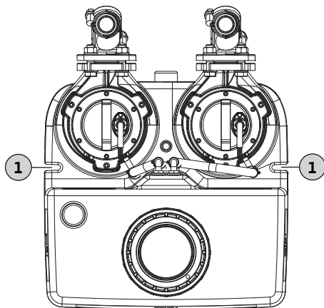
Fig. 2: Изглед отгоре на система за повишаване на налягането
