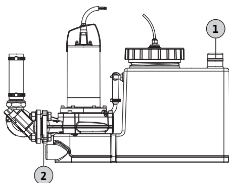
Fig. 6: Gyűjtőtartály légtelenítő csatlakozása
