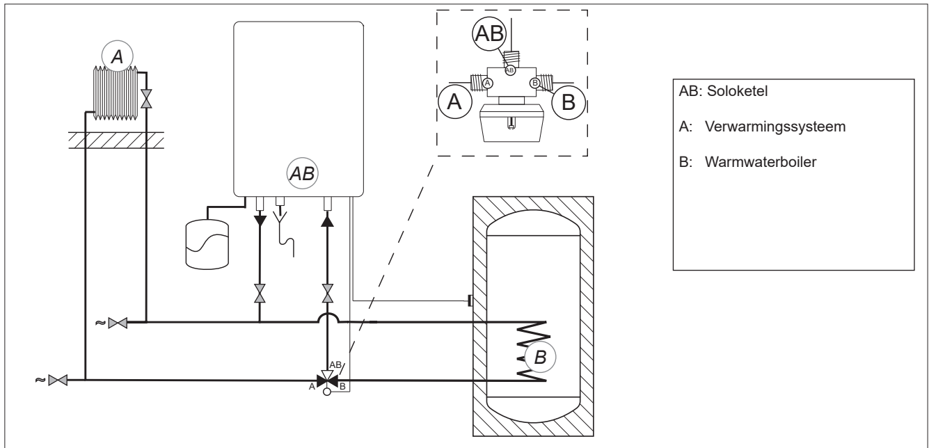
Hydraulisch schema met externe boiler
