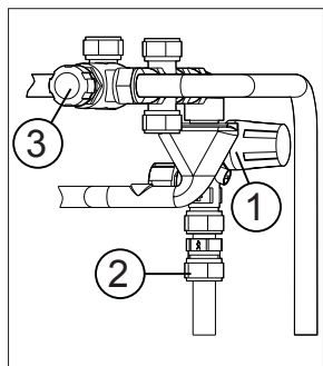
thermostatisch mengventiel, inlaatcombinatie en doseerventiel figuur 6.8.a
