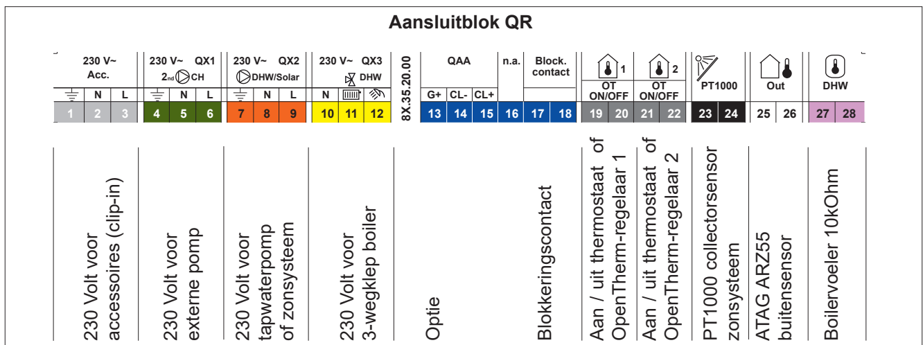
Aansluitblok
