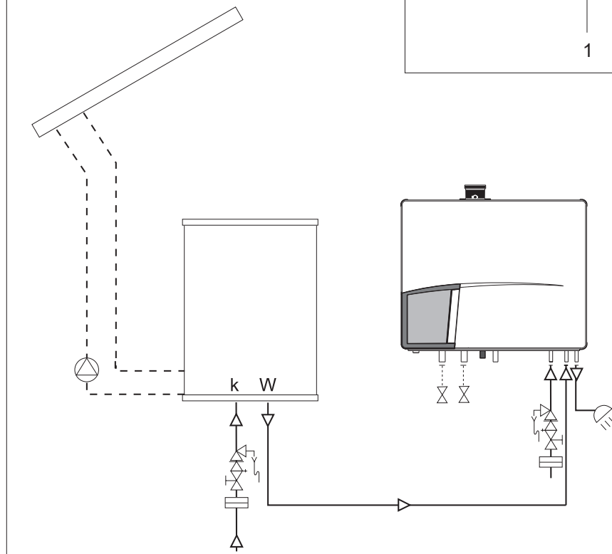
ATAG QR Combi met zonneboiler
