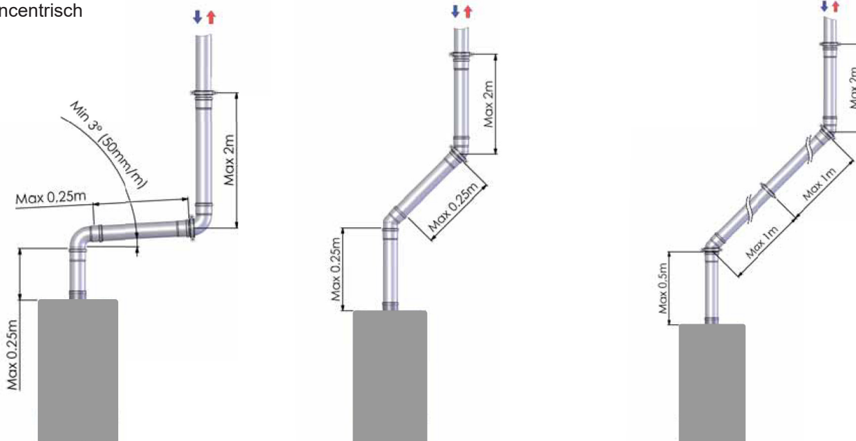
Beugelafstanden bij concentrisch aangesloten rookgasafvoer en luchttoevoer
