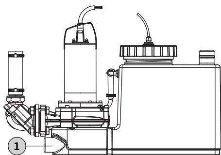
Fig. 7: Свързване на ръчна мембранна помпа
