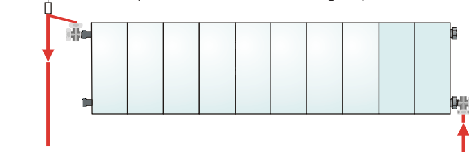
Verrohrung wechselseitig (bis zu 10 Kollektoren möglich)
