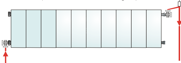
Verrohrung wechselseitig (bis zu 10 Kollektoren möglich)
