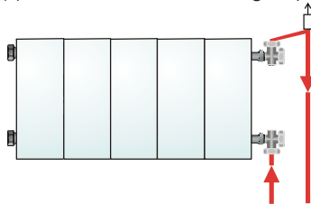
Verrohrung wechselseitig (bis zu 10 Kollektoren möglich)
