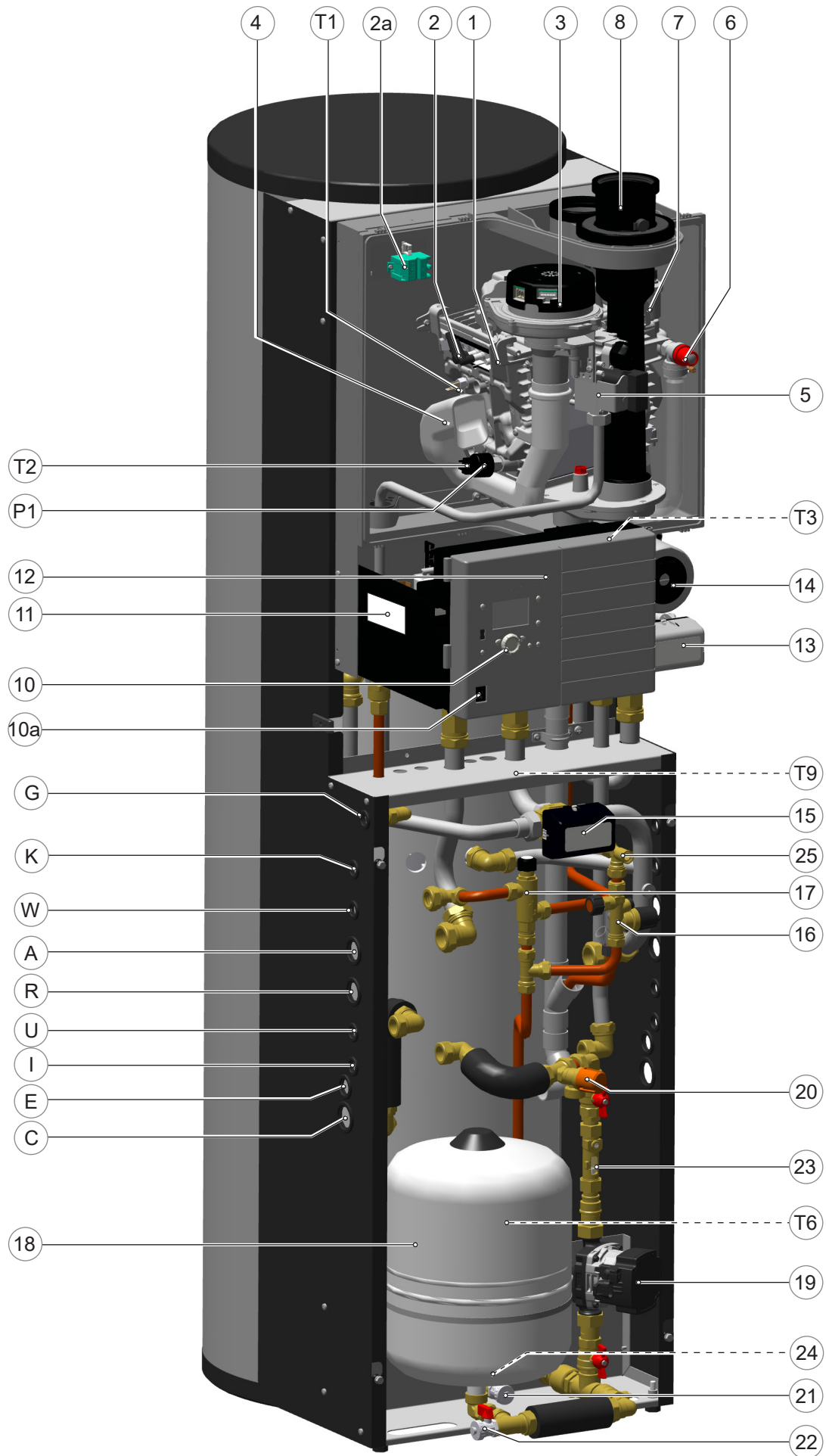
schematische ketelweergave ATAG QR-Solar Q25SCR200N Druksysteem
