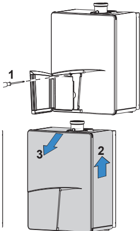
Mantel verwijderen
