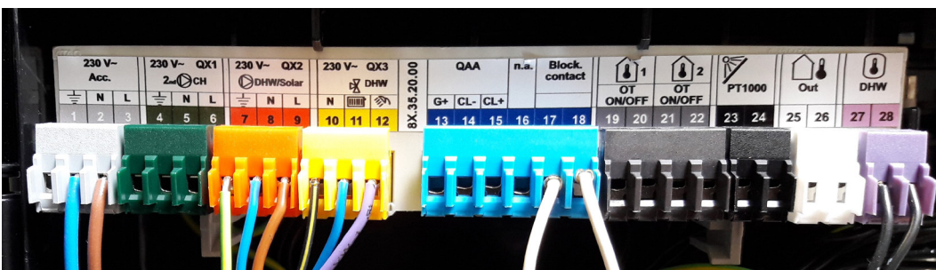
Aansluitblok
