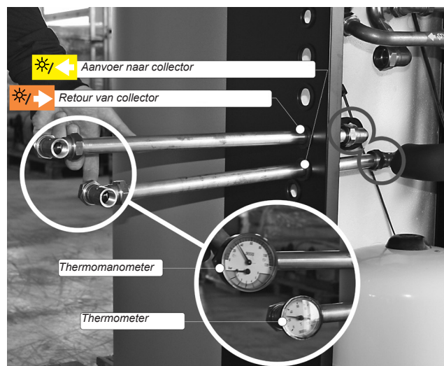
Collectoraansluitleidingen
