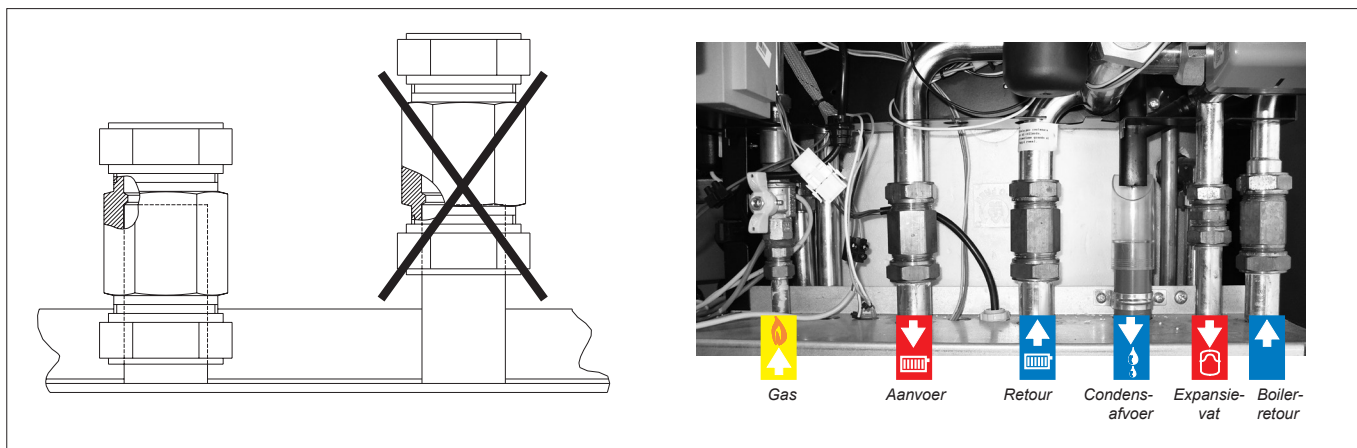
plaatsing schuifkoppelingen
