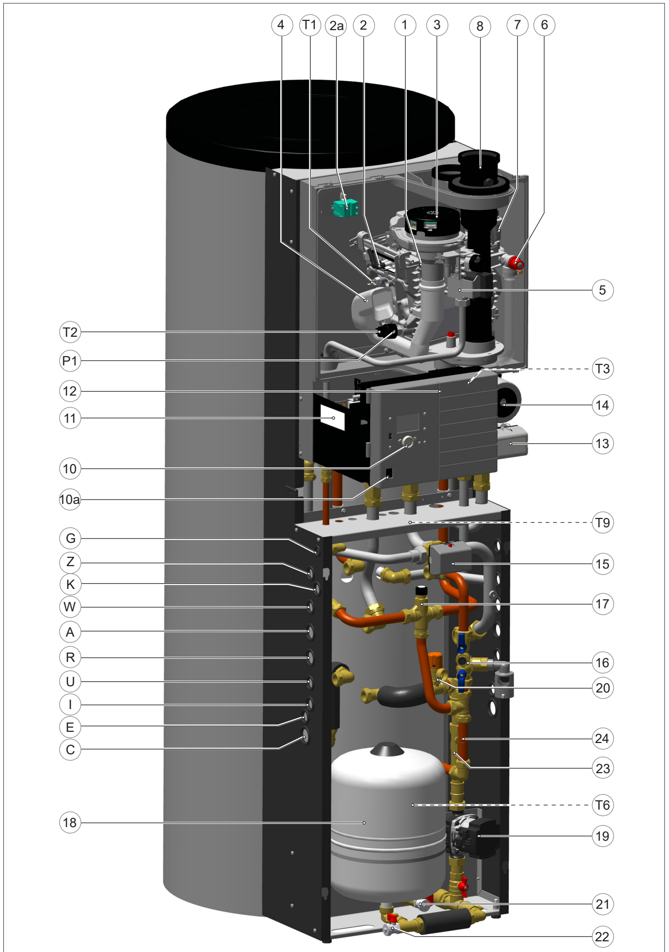
schematische ketelweergave ATAG QR-Solar Q38SCR380N Druksysteem
