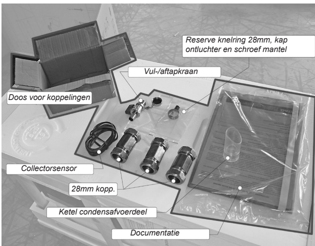
Leveringspakket bij de ketel (colli 2)
