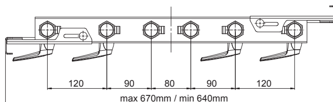
zijwandmontage
