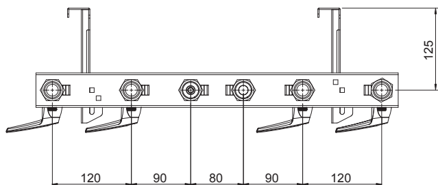
achterwandmontage
