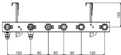
Achterwandmontage
