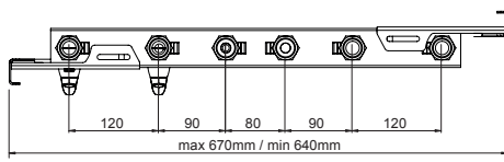
Zijwandmontage
