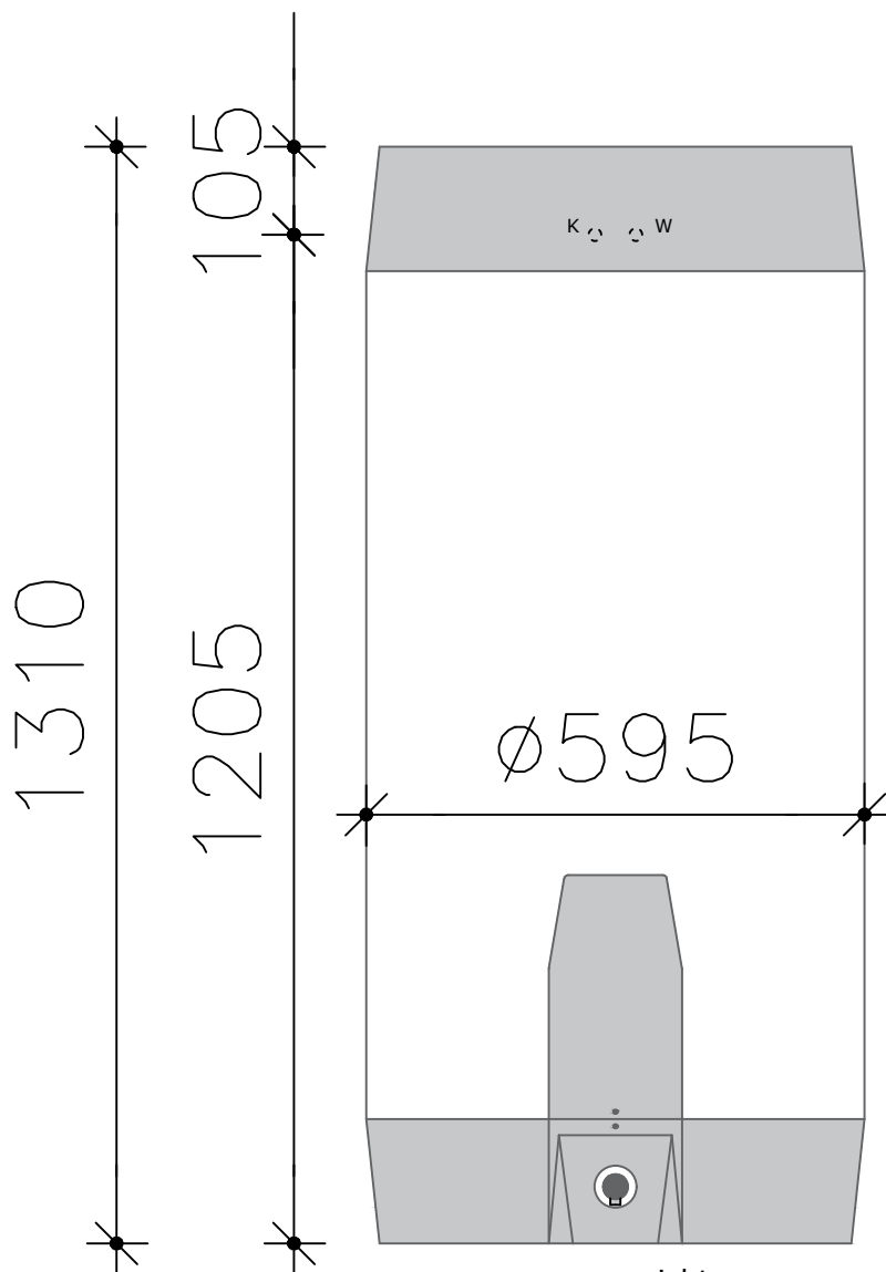
vooraanzicht
