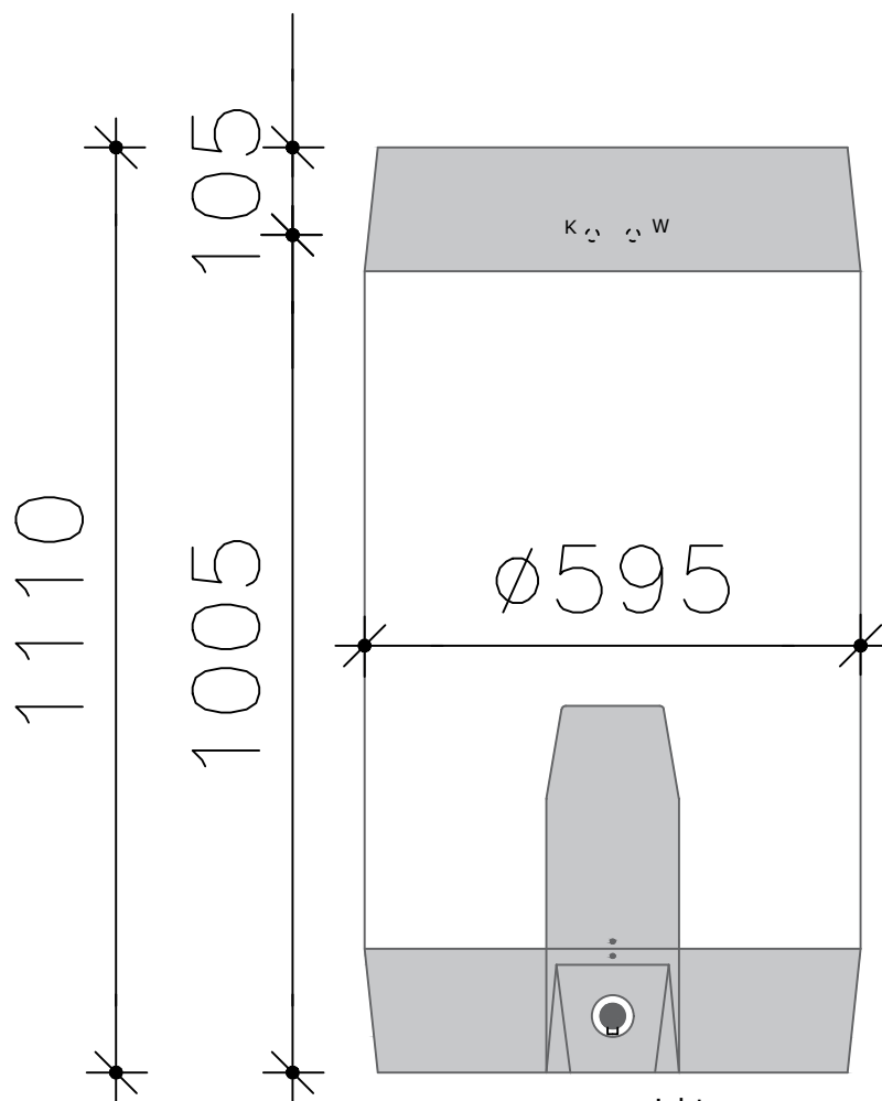
vooraanzicht
