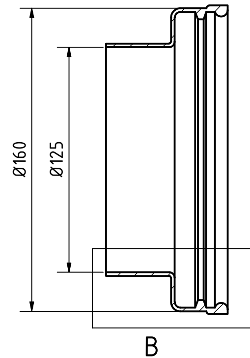
A-A ( 1 : 2 )
