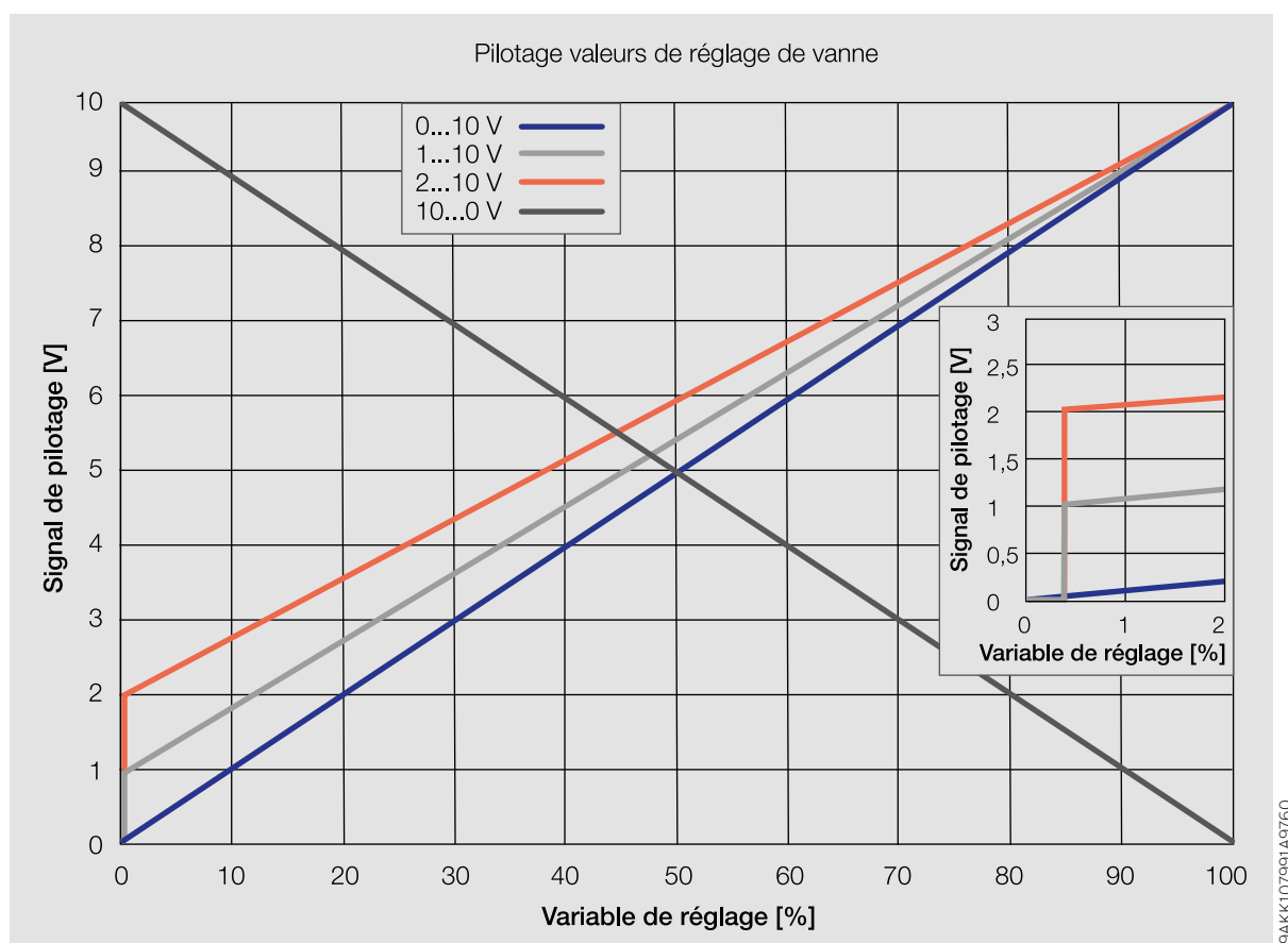
Fig. 34: Pilotage valeurs de réglage de vanne
