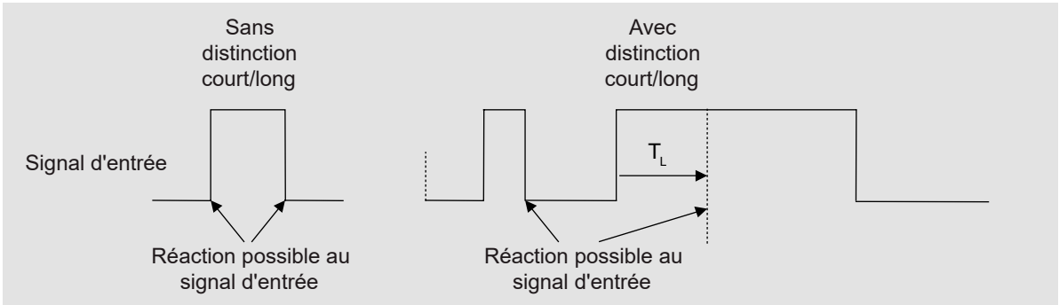
Fig. 27: Distinction entre appui long et court
