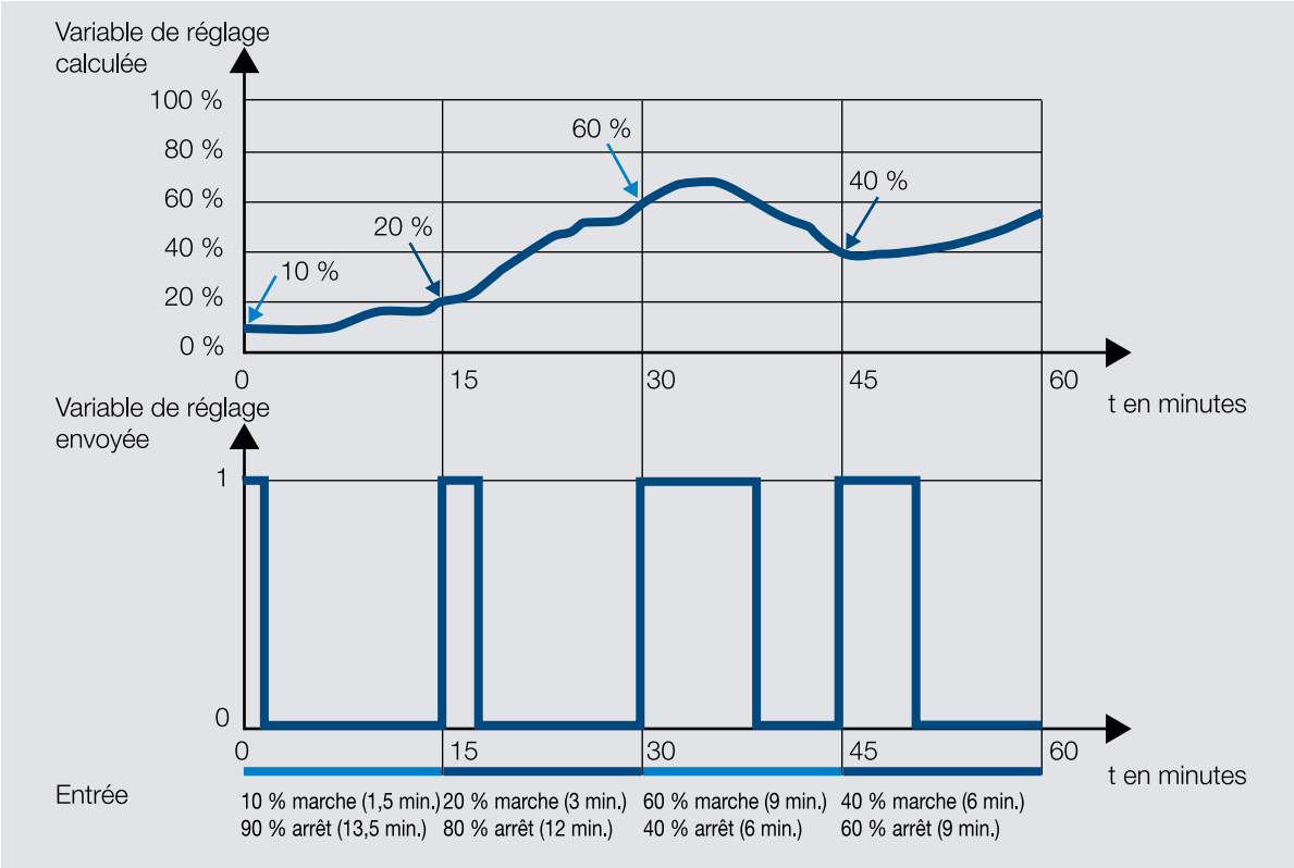
Fig. 33: Modulation de largeur d'impulsion - Exemple
