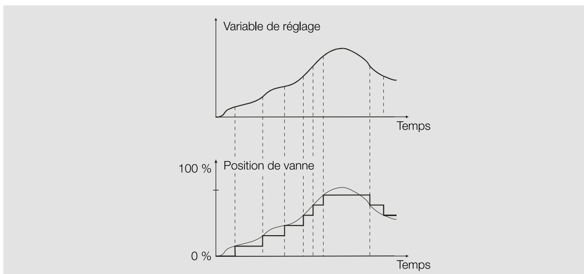
Fig. 30: Régulation continue
