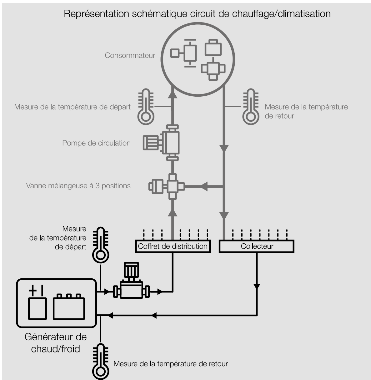
Fig. 36: Générateur de chaud/froid dans un circuit de chauffage/climatisation
