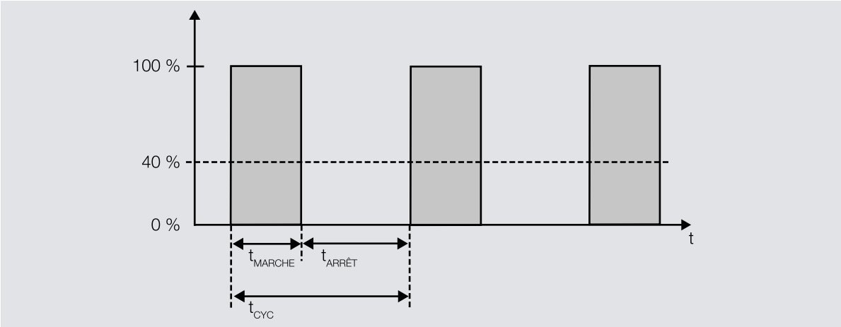
Fig. 32: Pilotage au moyen d'un rapport impulsion-pause variable
