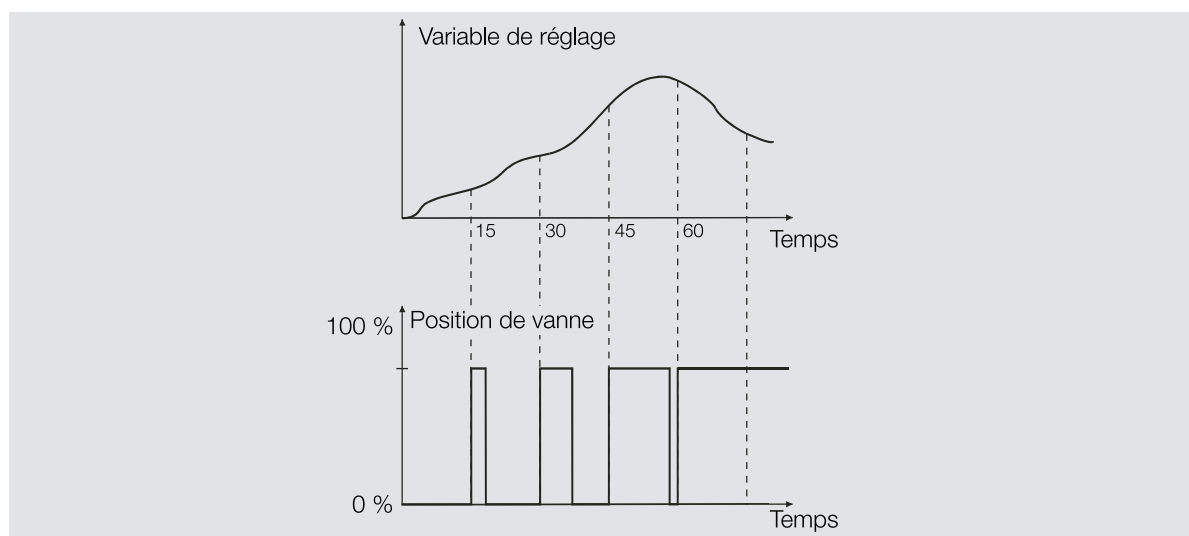
Fig. 31: Modulation de largeur d'impulsion (MLI)
