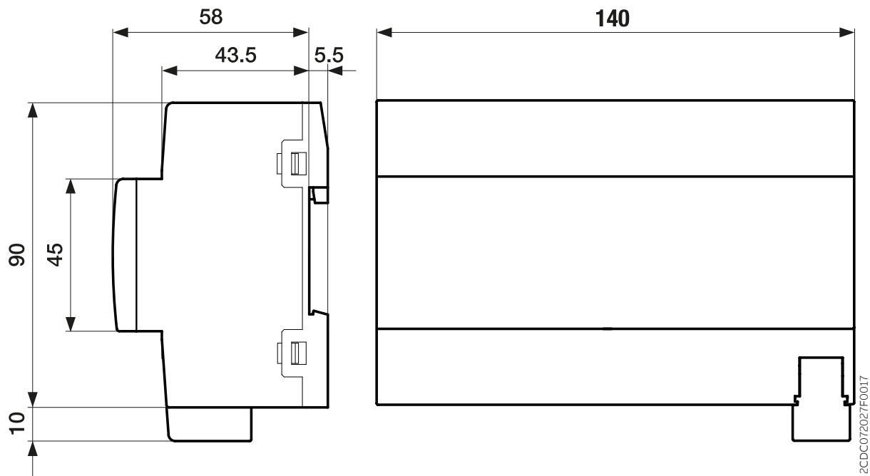
Fig. 11: Plan coté
