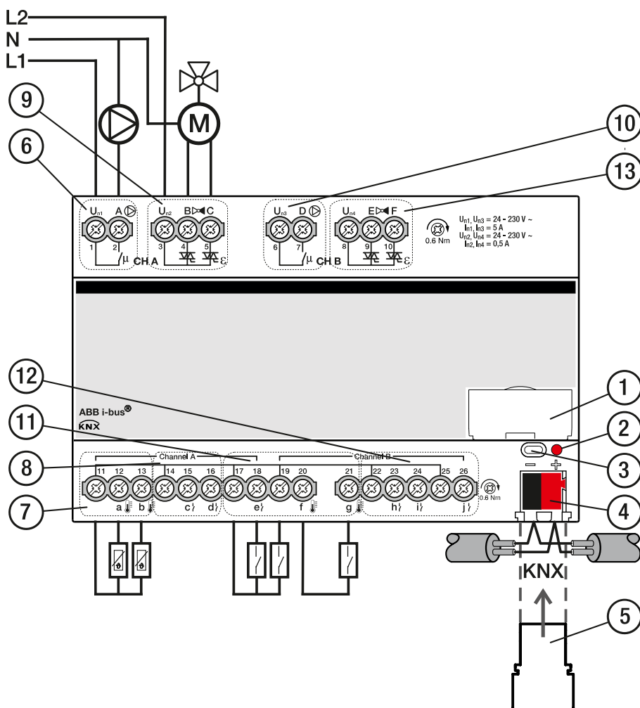
Fig. 9: Schéma de raccordement HCC/S 2.2.1.1
