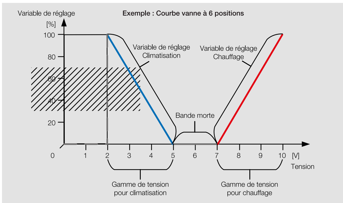
Fig. 35: Pilotage d'une vanne à 6 positions
