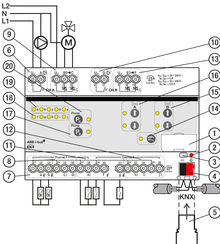
Fig. 12: Schéma de raccordement HCC/S 2.2.2.1
