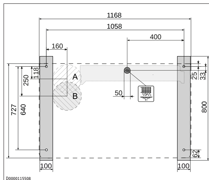
A Hydraulische aansluitingen met condensaatbak
