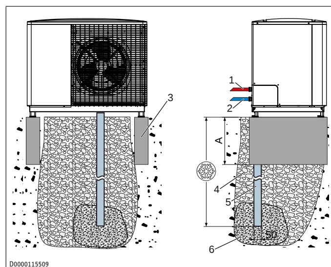
A Hydraulische aansluitingen met condensaatbak
