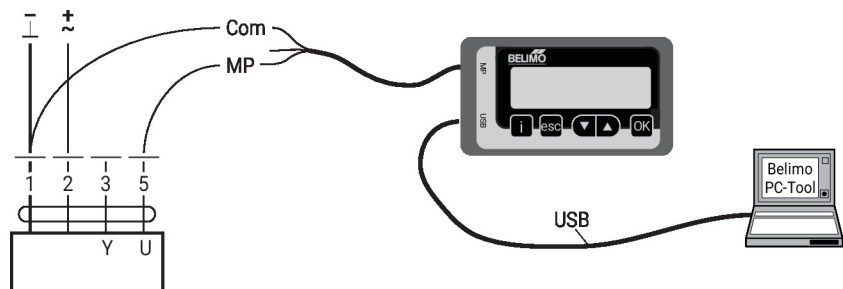
Anschluss PC-Tool
