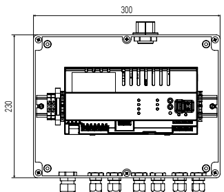
Maßzeichnungen, Angaben in mm
