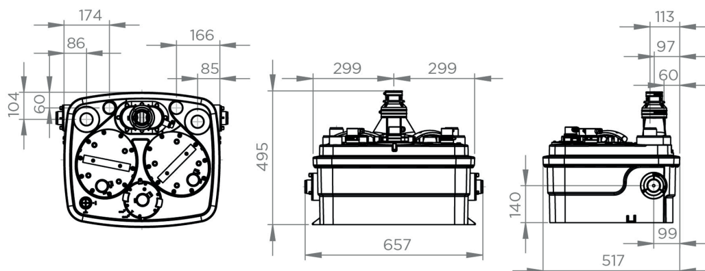
Afmetingen (mm)
