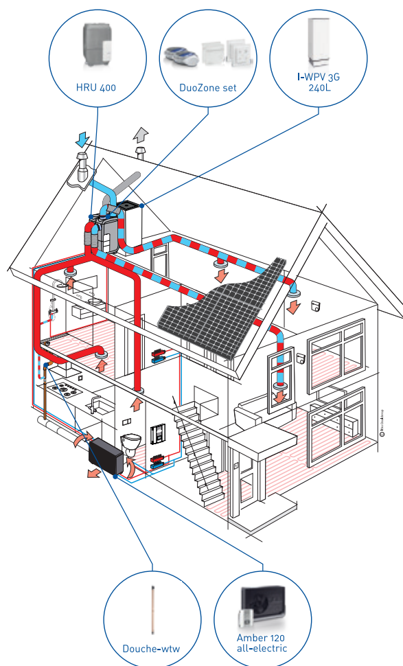
Amber 120 in een all-electric opstelling
