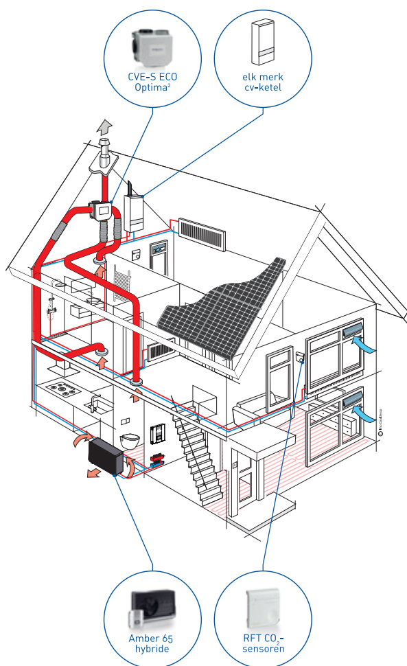
Amber 65 in een hybride opstelling
