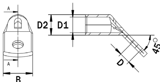
45° angle cable lugs
