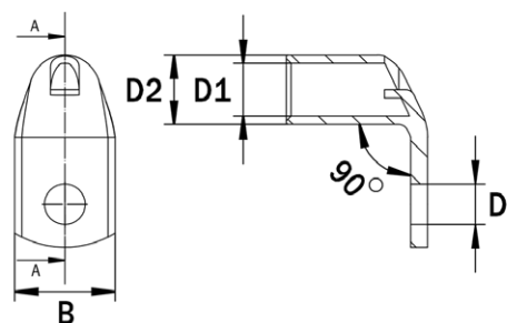
90° angle cable lugs
