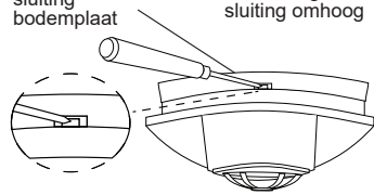
figuur 3 Beveiligde sluiting bodemplaat Druk met een schroevendraaiër de beveiligde sluiting omhoog
