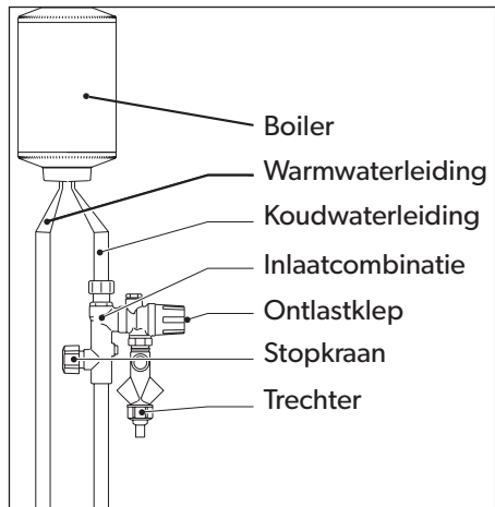
Figuur 3 Principewerking
