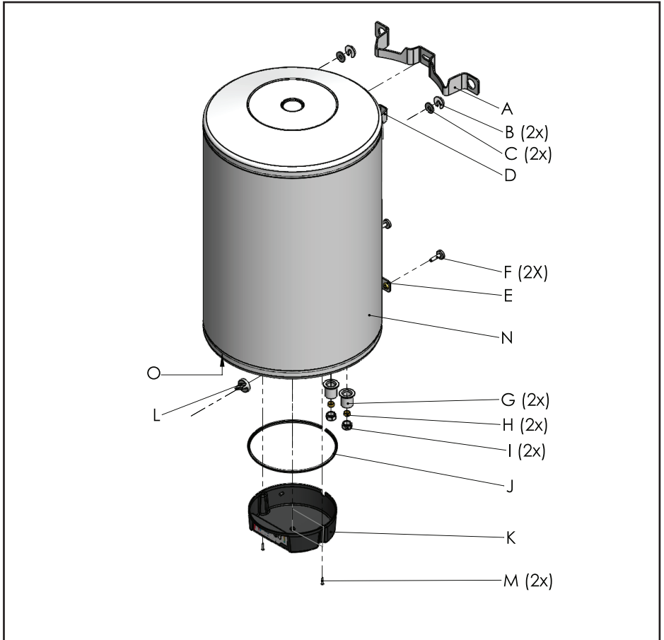
Illustration 1 Composants principaux
