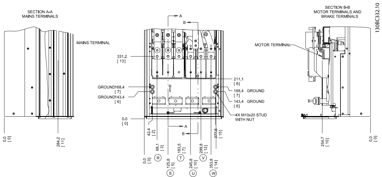
Kuva 4.6 Liitinten paikat, D2h
