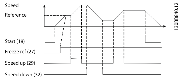
Kuva 6.1 Nopeus ylös/alas
