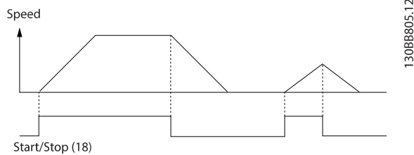
Kuva 6.2 Käynnistys-/pysäytyskomento STO-toiminnolla
