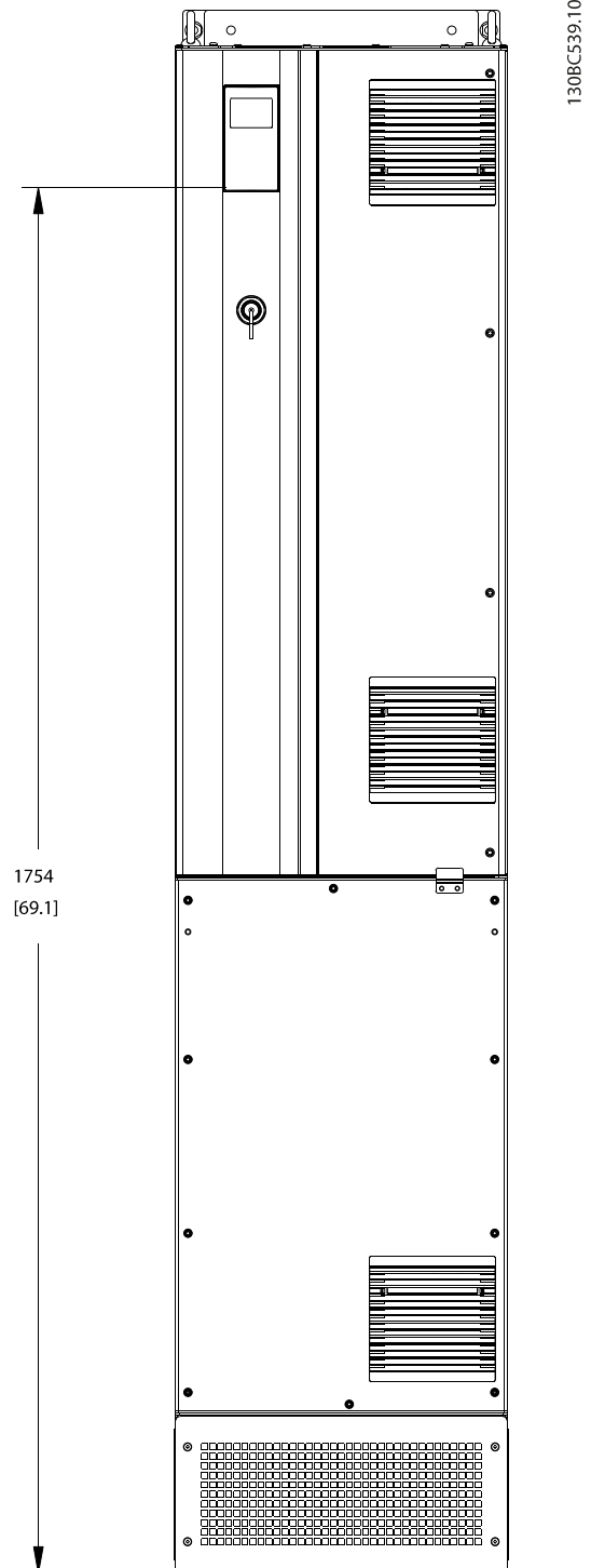
Kuva 1.2 D7h Kotelointi
