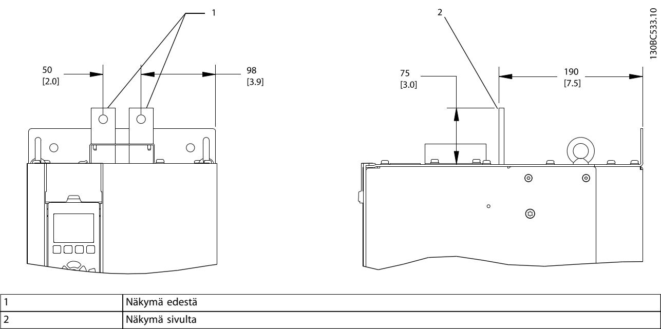
Kuva 4.8 Kuormituksenjako- ja regenerointiliittimet, D3h
