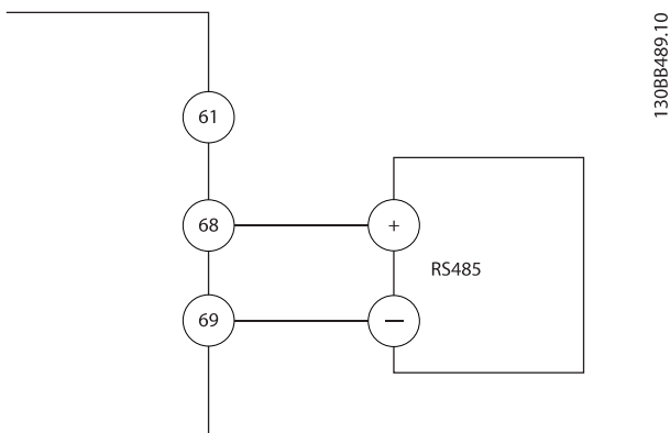
Kuva 4.28 Sarjaliikenteen kytkentäkaavio
