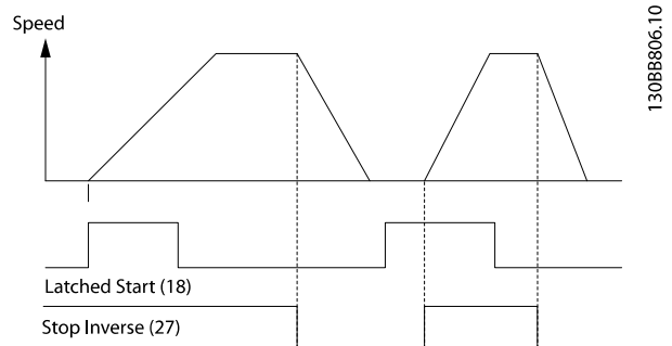
Kuva 6.3 Pulssikäynnistys/pysäytys käänteinen
