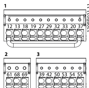
Obrázek 4.25 Čísla svorek
