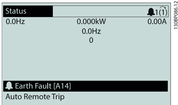
Slika 7.2 Primer alarma
