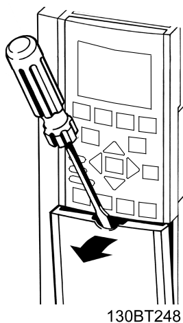
Slika 4.4 Pristup ožičavanju za kućišta IP20 i IP21
