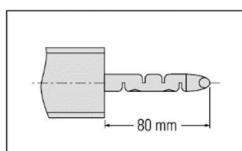
B Gelede testvinger, (L = 80 mm, Ø 12 mm). Testkracht 10 N.
