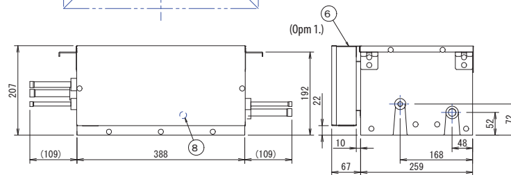
Plaats van het naamplaatje van de unit ••• Rechts van de schakelkast
