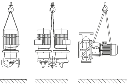
Fig. 1: Přeprava čerpadla
