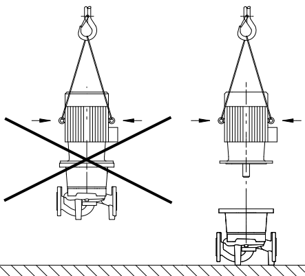
Fig. 2: Přeprava motoru
