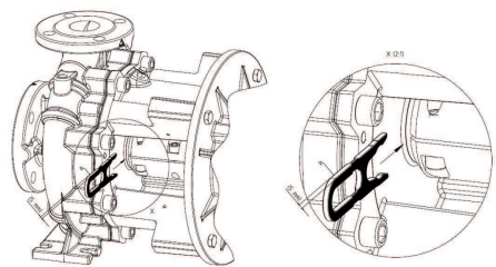
Fig. 47: Nasazení montážního rozpidleného klíče
