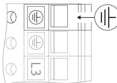
Fig. 28: Dodatečné uzemnění, od výkonu motoru 11 kW
