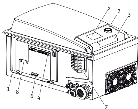
Fig. 5: Elektronický modul, přehled
