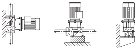
Fig. 3: Vaade Stratos GIGA
