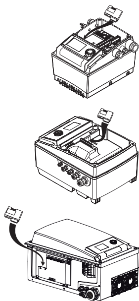
Fig. 10: IF-mooduli paigaldamine
