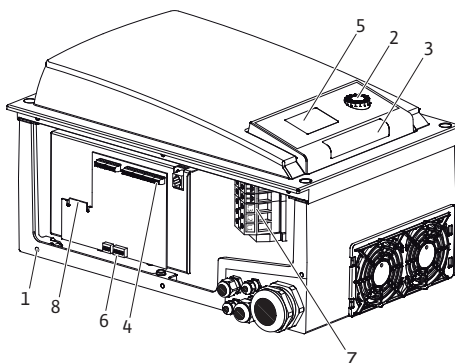
Fig. 5: Elektroonikamoodul, ülevaade
