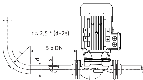
Fig. 18: Summutusala pumba ees ja järel
