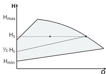
Fig. 7: Reguleerimisviis \Delta p-v
