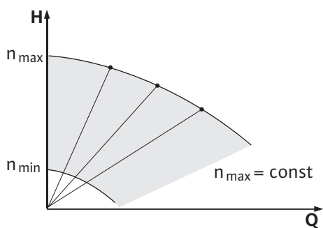
Fig. 33: Режим управления
