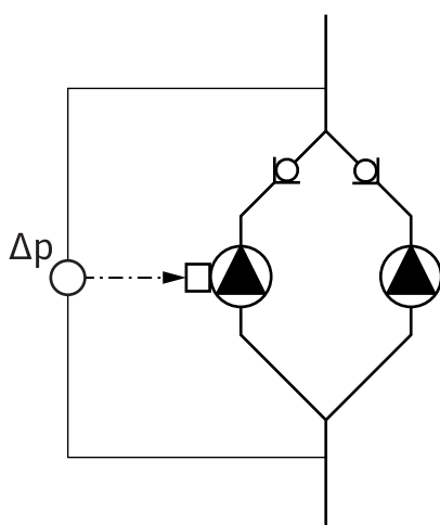
Fig. 9: Пример: подсоединение дифференциального датчика давления в установке разветвленной трубы
