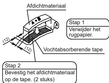
Afb. 1 Luchtuitlaat
