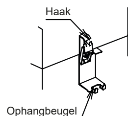
Afb. 5 Na installatie
