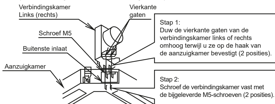
Afb. 7 Installatie van verbindingkamer (deze afbeelding toont de linkse verbindingkamer.)
