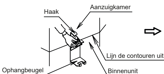
Afb. 4 Installatie
