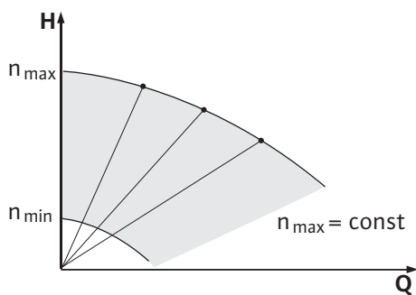
Fig. 33: Режим керування
