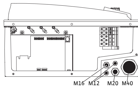
Fig. 29: Кабельні нарізні з'єднання
