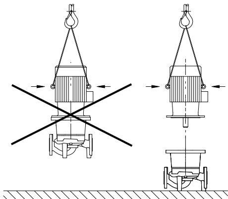
Fig. 2: Транспортування двигуна
