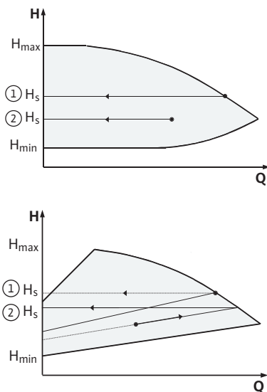
Fig. 32: Регулювання \Delta p -с/ \Delta p -v
