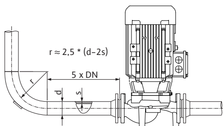
Fig. 18: Дільниця, на якій відбувається вирівнювання потоку, перед насосом та за ним
