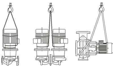
Fig. 1: Транспортування насоса
