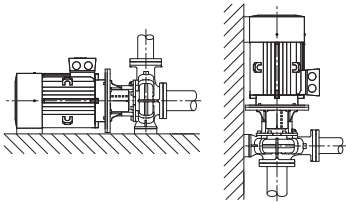
Fig. 4: Вигляд Stratos GIGA B
