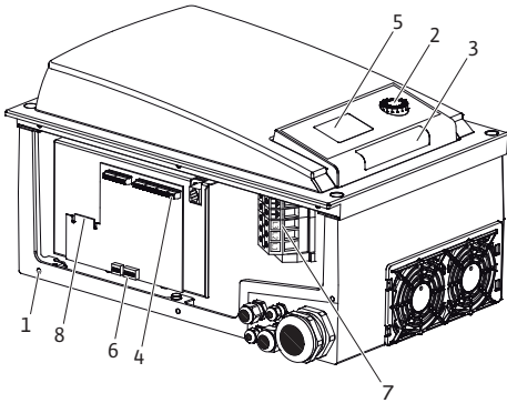
Fig. 5: Електронний модуль, огляд
