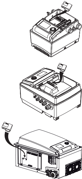
Fig. 10: Застосування IF-модуля
