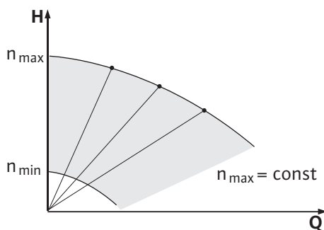
Fig. 8: Режим керування
