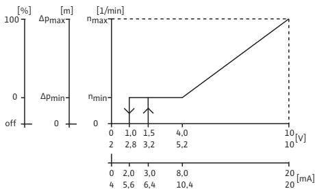
Fig. 12: Функціонування входу і виходу
