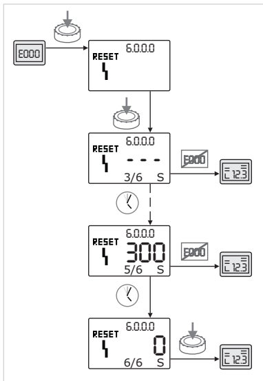
Fig. 56: Квитування помилок типу C
