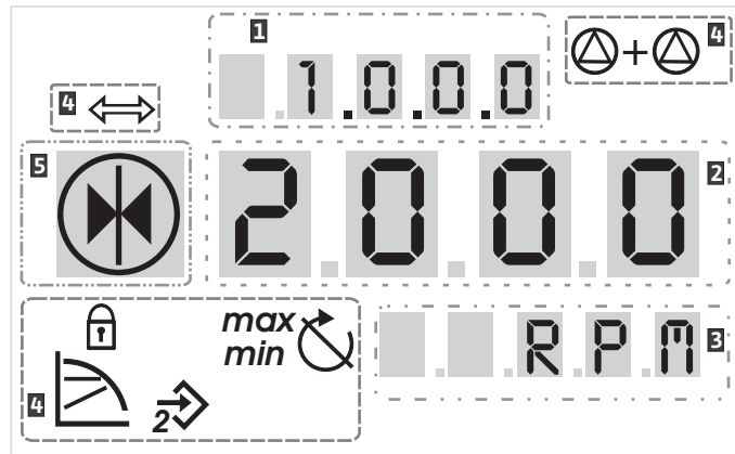
Fig. 36: Структура дисплея
