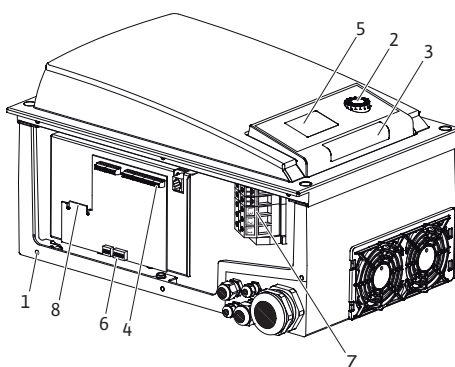
Fig. 5: Elektronikkmodul, oversikt
