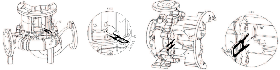
Montasjegaffel for innstillingsarbeid
