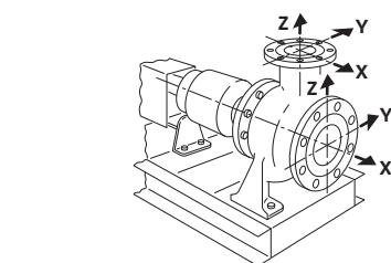
Fig. 22: Belastningstype 1A
