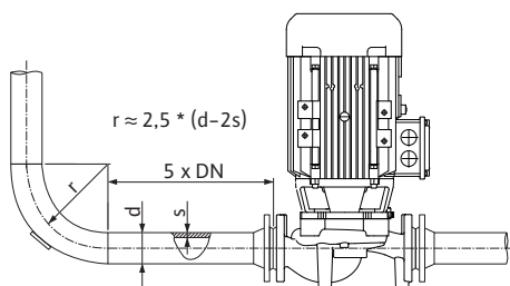
Fig. 18: Hvilestreking før og etter pumpen
