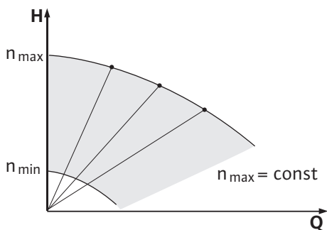
Fig. 8: Manuell drift
