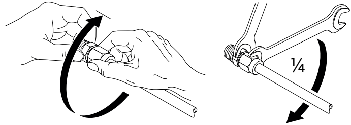
Fig. 19: Dreie klemringskrutilkoblingen 1/4 omdreining til
