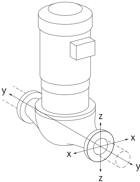
Fig. 20: Belastningstype 16A, EN ISO 5199, vedlegg B
