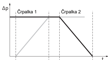
Fig. 11: Preklop črpalck, shematični
