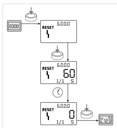
Fig. 51: Potrditev tipa napake A ali D
