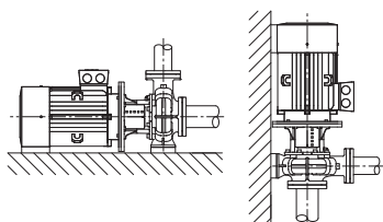
Fig. 4: Prikaz črpalke Stratos GIGA B
