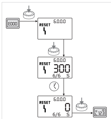
Fig. 54: Potrditev tipa napake B ( X=Y )
