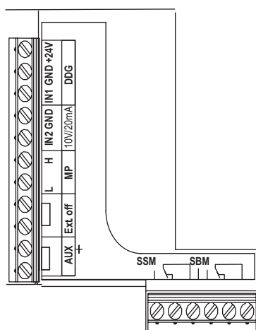
Fig. 26: Krmilne sponke
