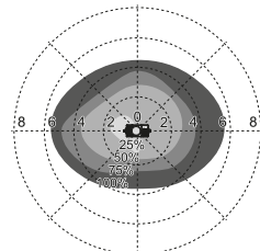
Ansprechbereich Deckenmontage (Einheit: m) Empfohlene Montagehöhe: 3m
