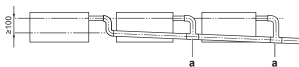
a T-stuk
