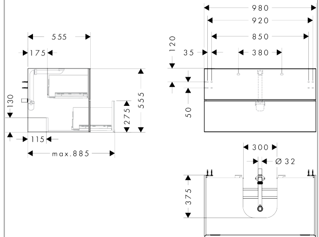
Maattekening
