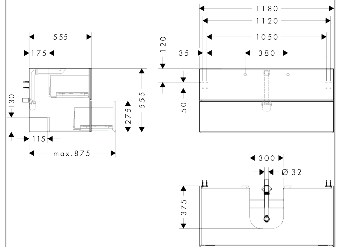
Maattekening
