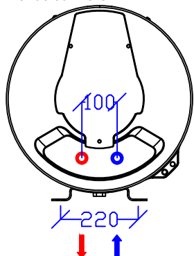
Onderaanzicht
